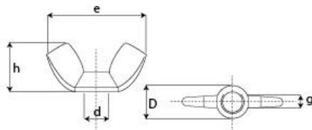
Гайка крилчата DIN 315, поцинкована, клас на якост 6
